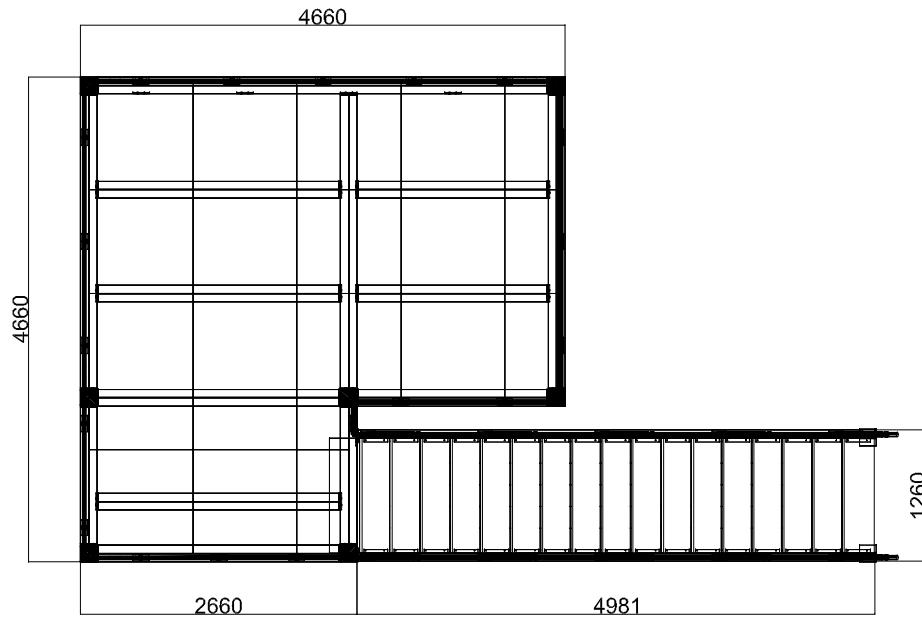
Grundriss
