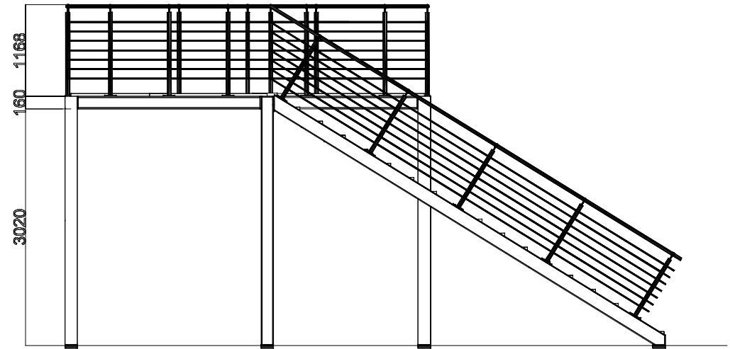
Seitenansicht
