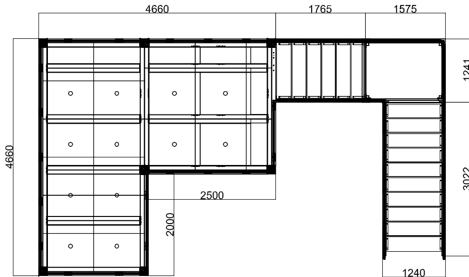
Grundriss
