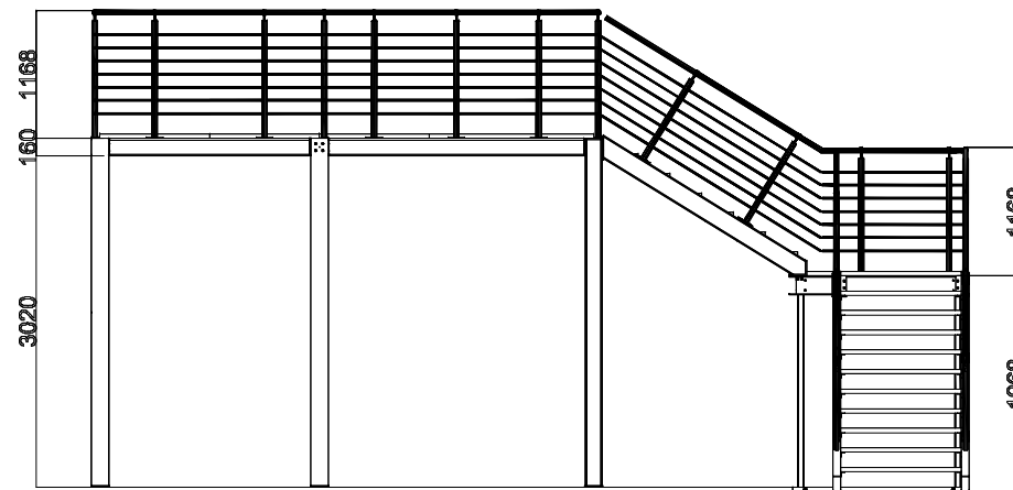
Seitenansicht
