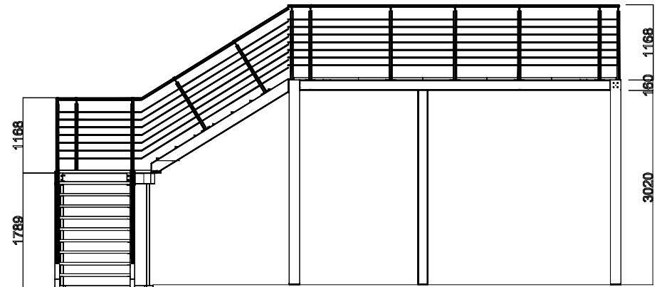
Seitenansicht
