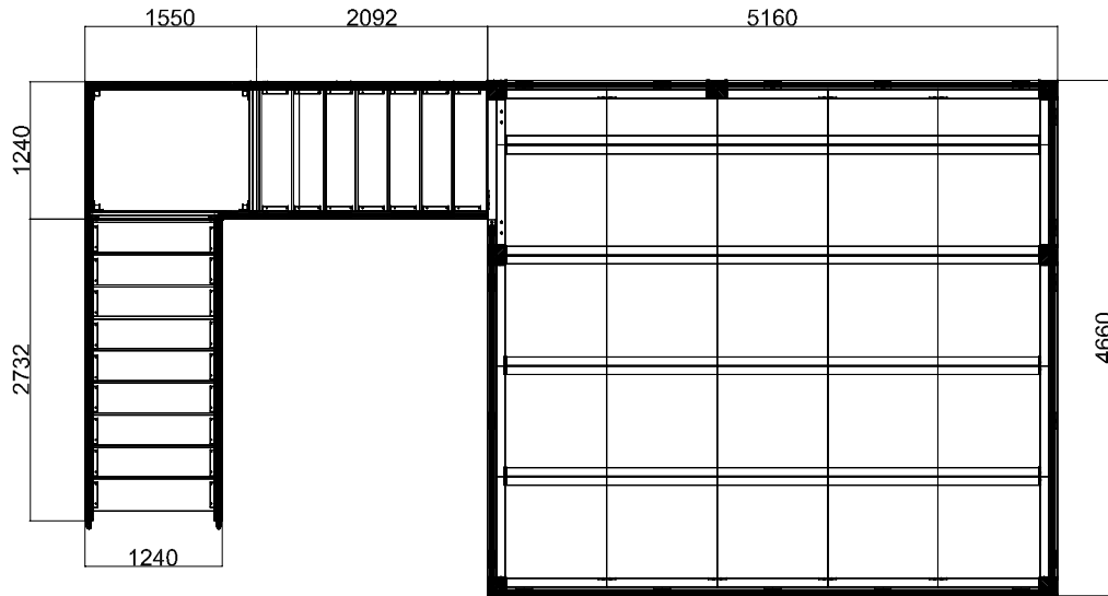
Grundriss
