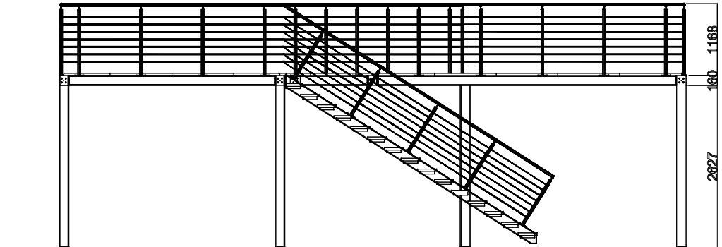
Seitenansicht
