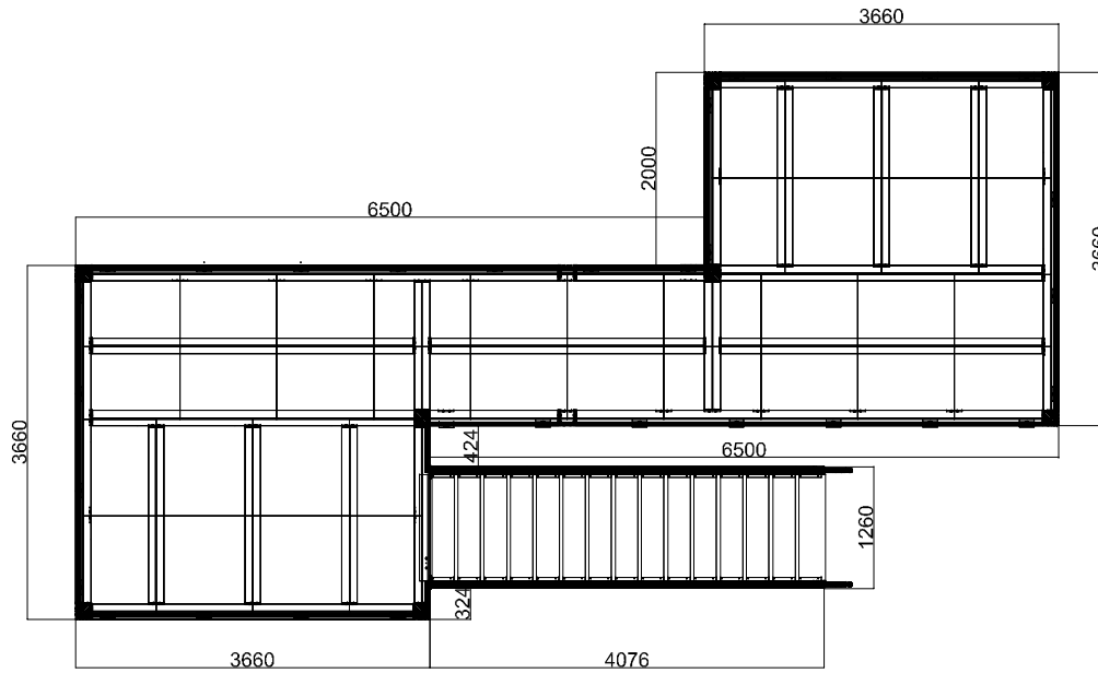
Grundriss
