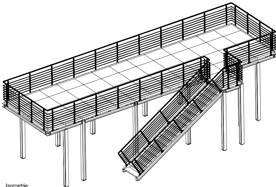
Isometrie
