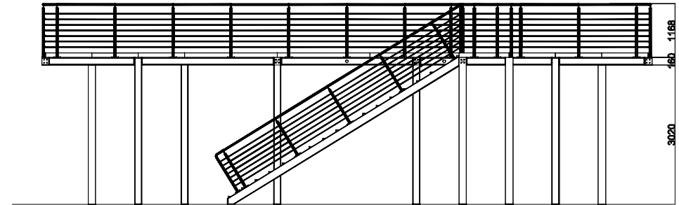
Seitenansicht
